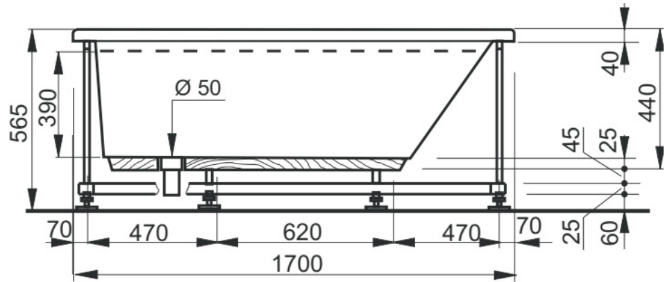
Presek "A-A"
