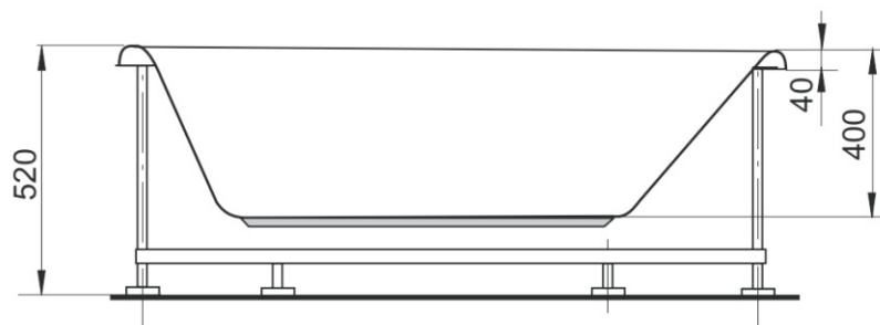
Presek "A-A"
