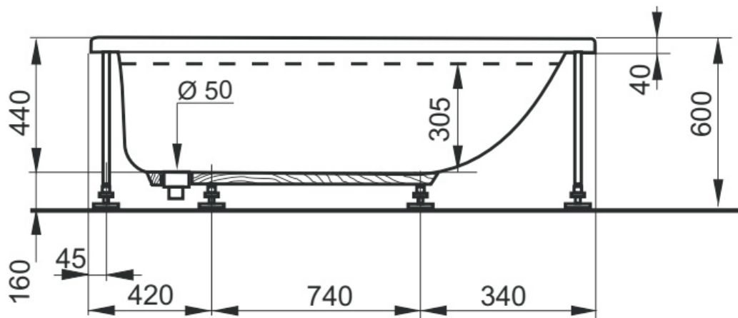
Presek "A-A"
