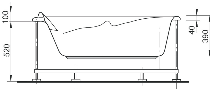
Presek "A-A"
