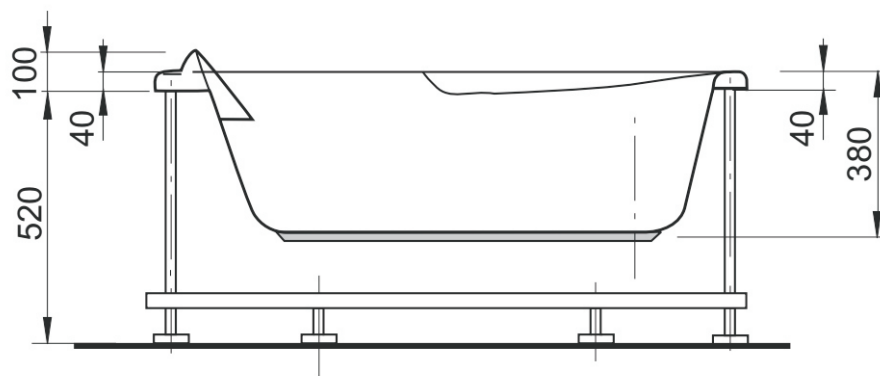
Presek "A-A"
