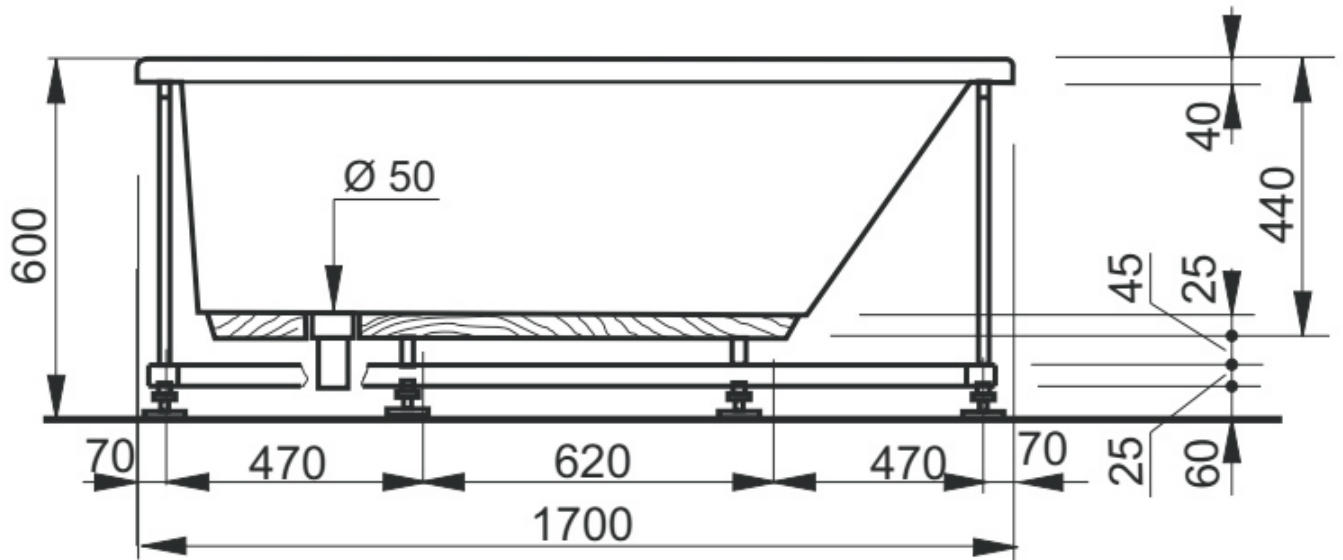
Presek "A-A"
