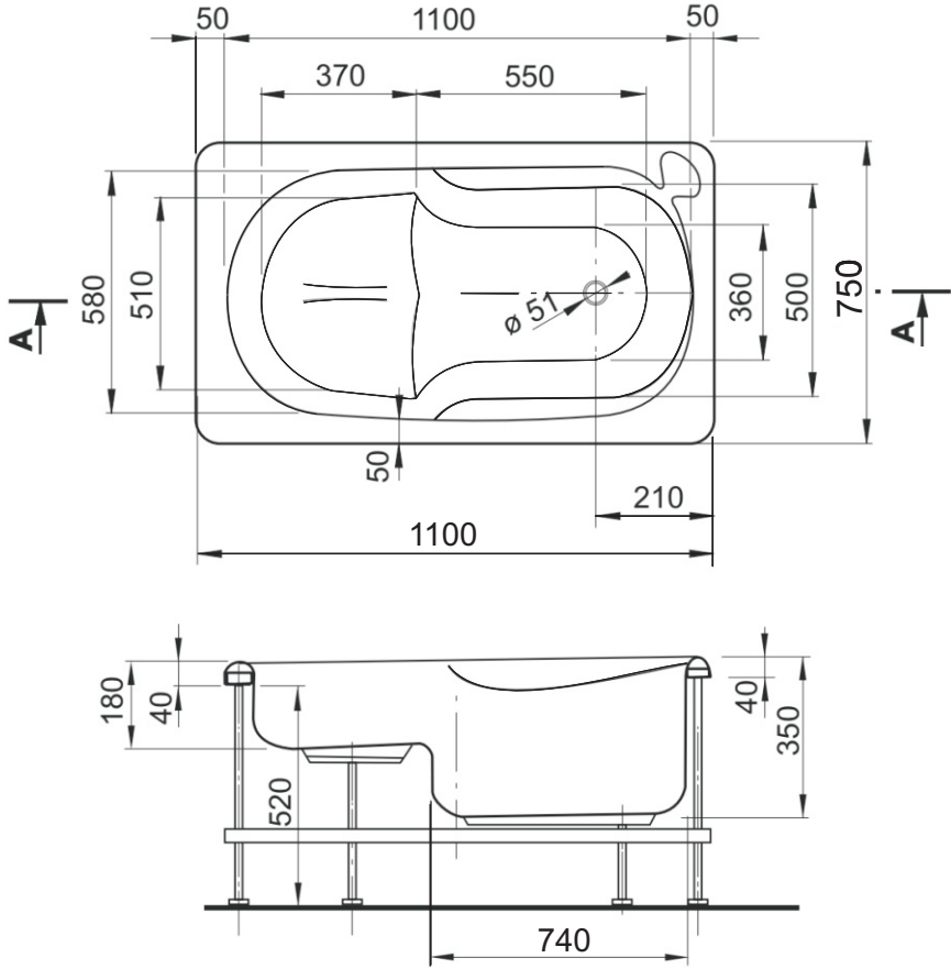
Presek "A-A"
