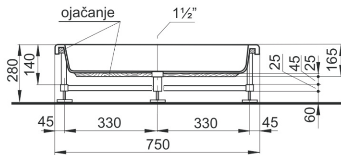
Presek "A-A"
