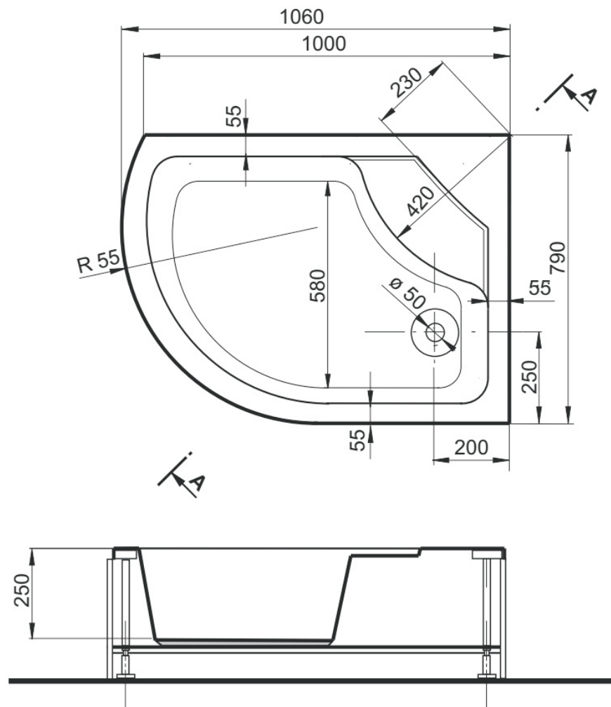
Presek "A-A"
