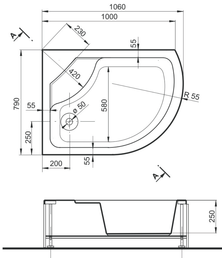
Presek "A-A"
