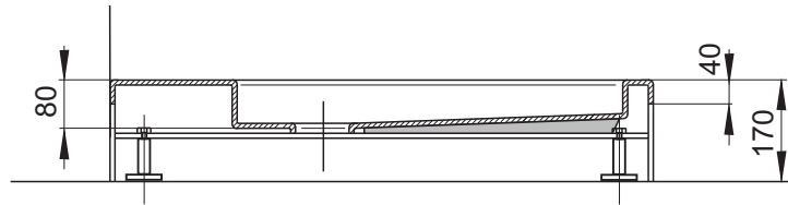
Presek "A-A"
