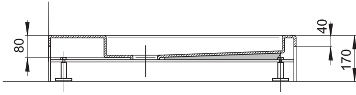
Presek "A-A"
