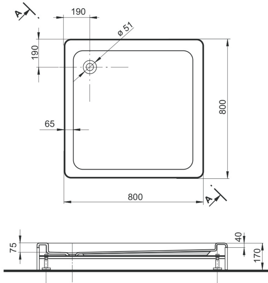
Presek "A-A"
