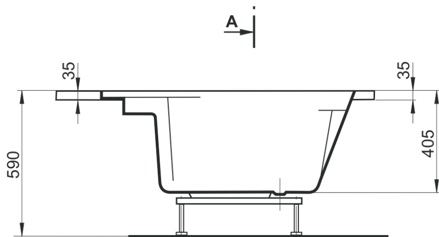
Presek "A-A"
